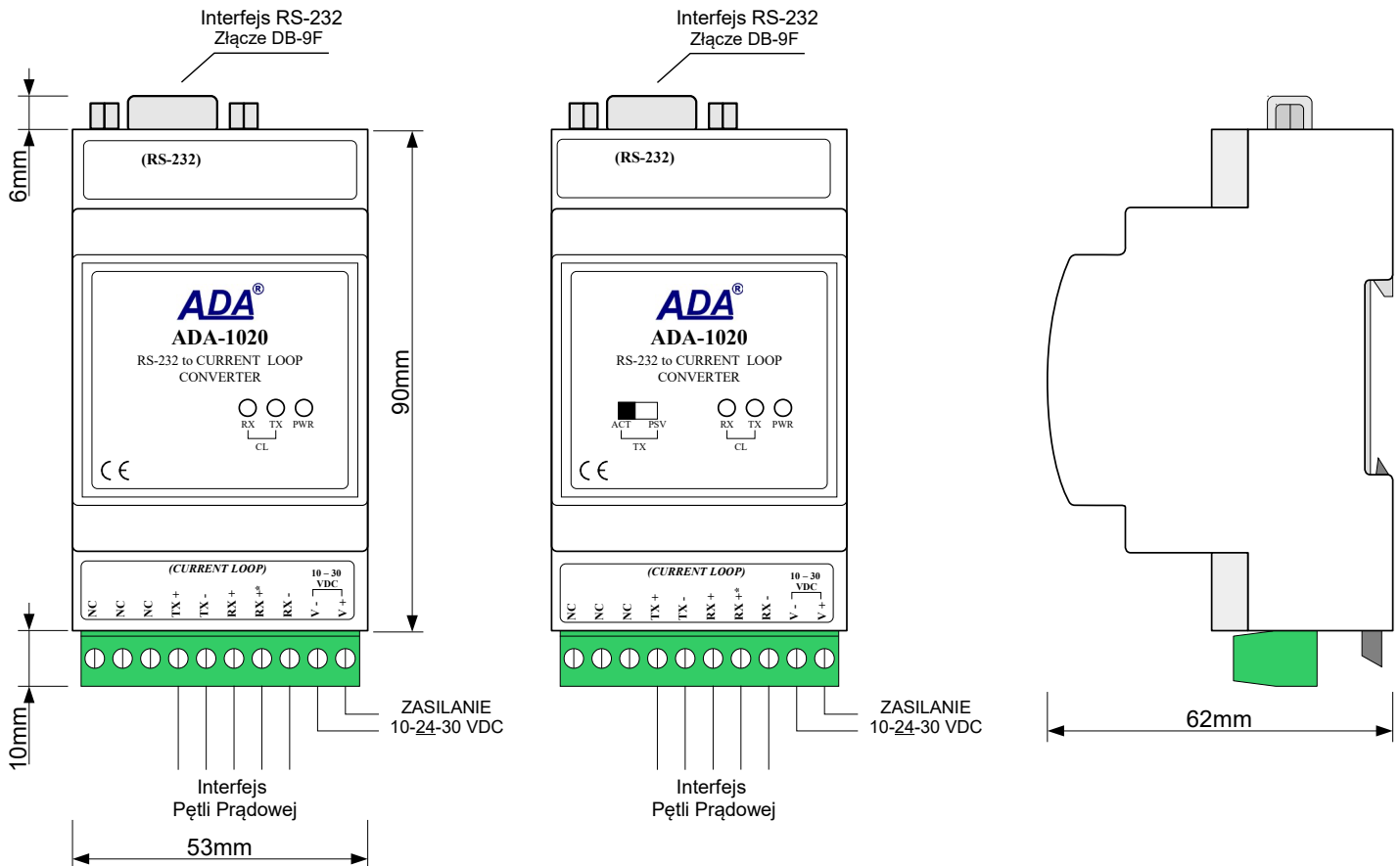
Wersja z aktywnym nadajnikiem +/- 20mA
