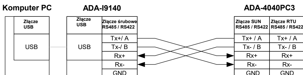
Rys 4. Podłączenie 4-przewodowe ADA-4040PC3 do komputera PC za pomocą konwertera USB na RS485/RS422 ADA-I9140
