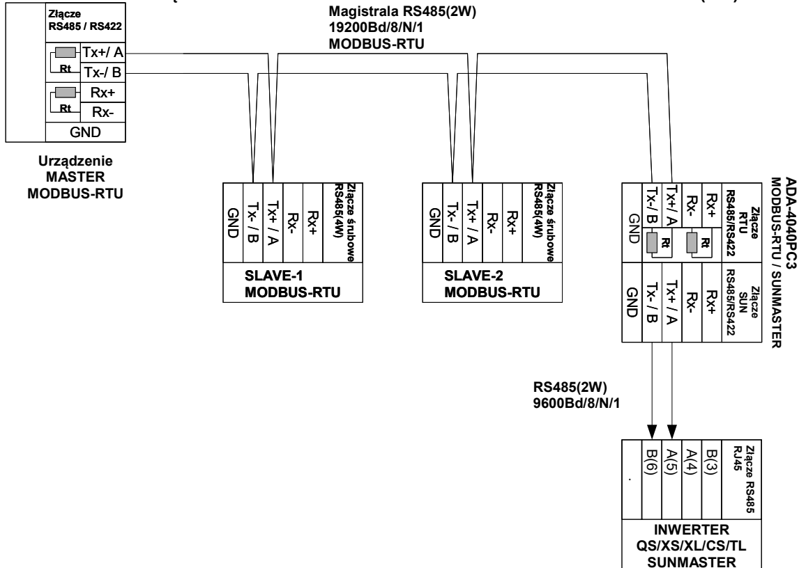
Rys 7. Przykładowe podłączenie ADA-4040PC3 do magistrali RS485(2W) 2-przewodowej oraz Inwertera SunMaster do ADA-4040PC3
