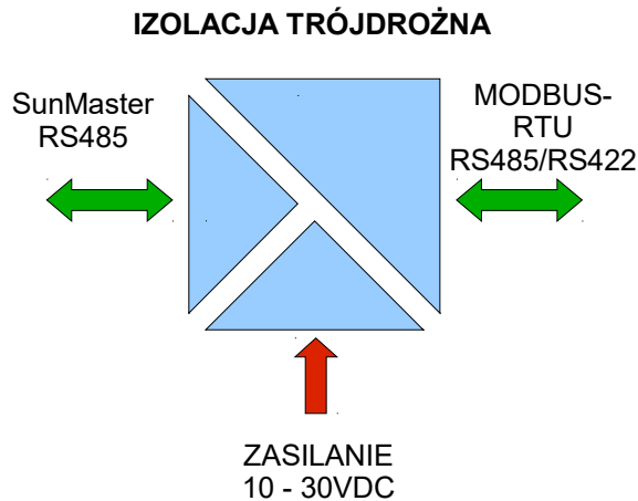
Rys 2. Struktura izolacji
