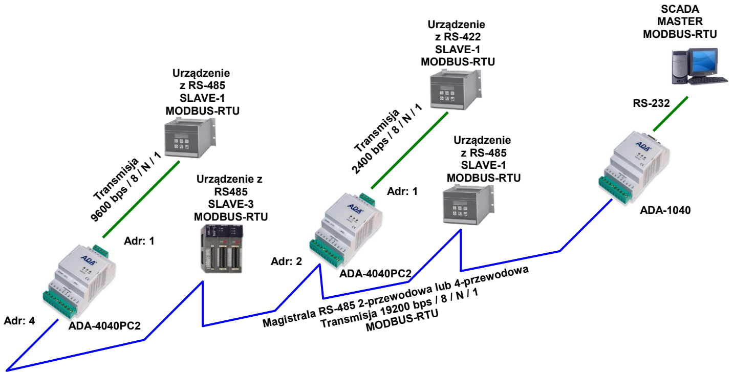
Rys 10. Podłączenie urządzeń MODBUS-RTU/JBUS o stałym adresie do magistrali RS485 MODBUS-RTU/JBUS
