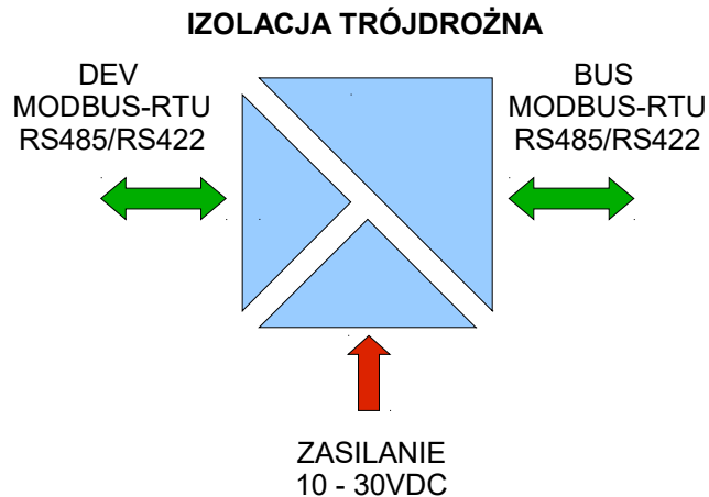
Rys 2. Struktura izolacji
