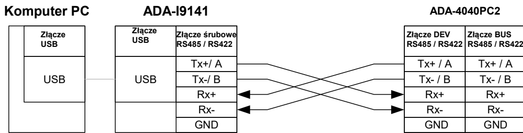
Rys 4. Podłączenie 4-przewodowe ADA-4040PC2 do komputera PC za pomocą konwertera USB na RS485/RS422 ADA-I9141
