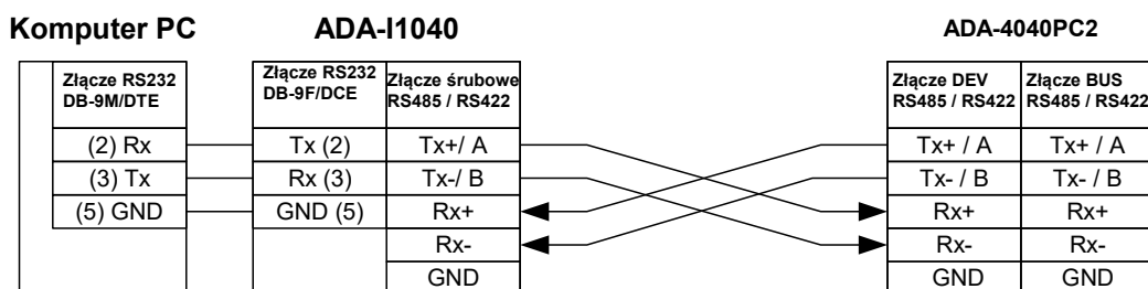
Rys 3. Podłączenie 4-przewodowe ADA-4040PC2 do komputera PC za pomocą konwertera RS232 na RS485/RS422 ADA-I1040
