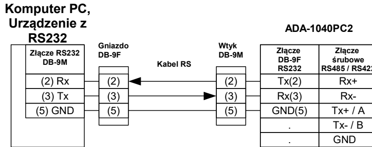
Rys 4. Podłączenie ADA-1040PC2 do komputera PC lub urządzenia z RS232 za pomocą kabla
