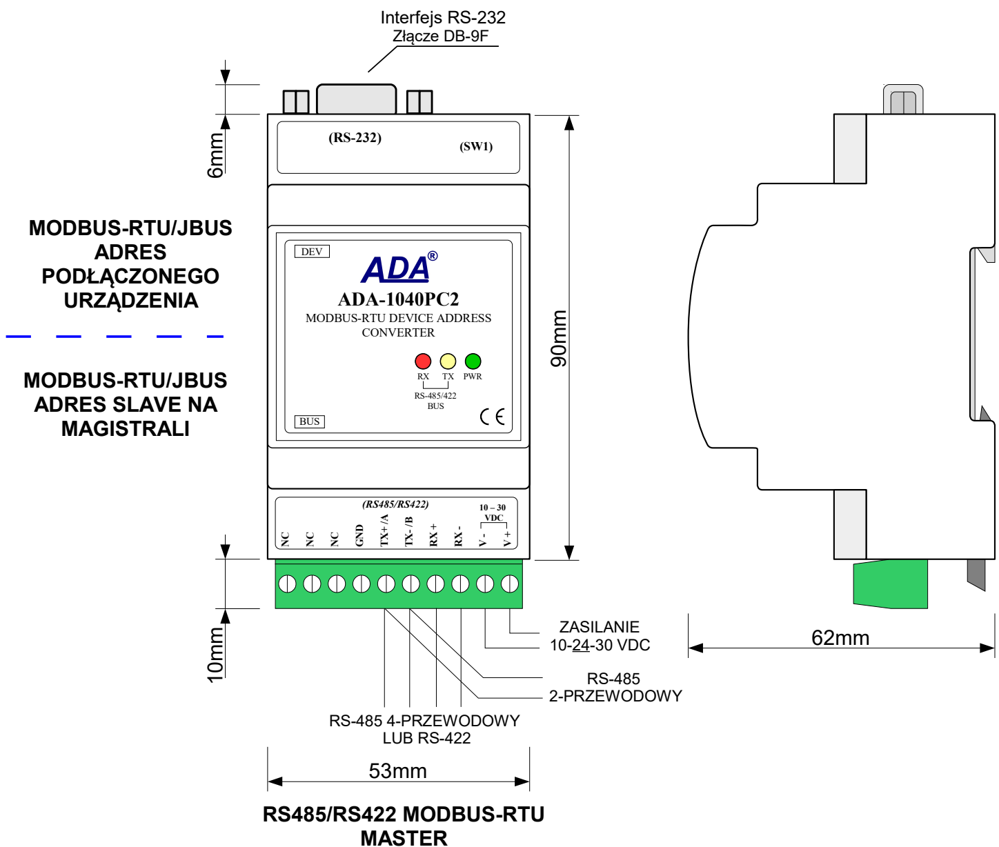
Rys 1. Widok ADA-1040PC2 oraz położenie przełącznika SW1
