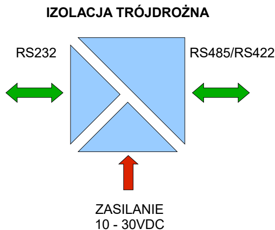
Rys 2. Struktura izolacji w ADA-1040PC2
