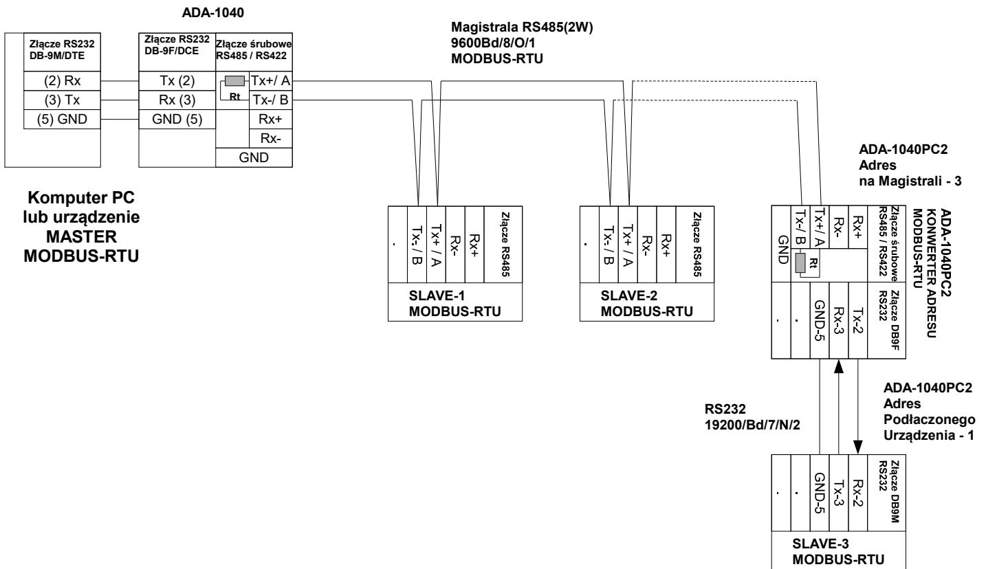
Rys 7. Przykładowe podłączenie ADA-1040PC2 do magistrali RS485(2W) 2-przewodowej oraz separacja galwaniczna urządzeń SLAVE
