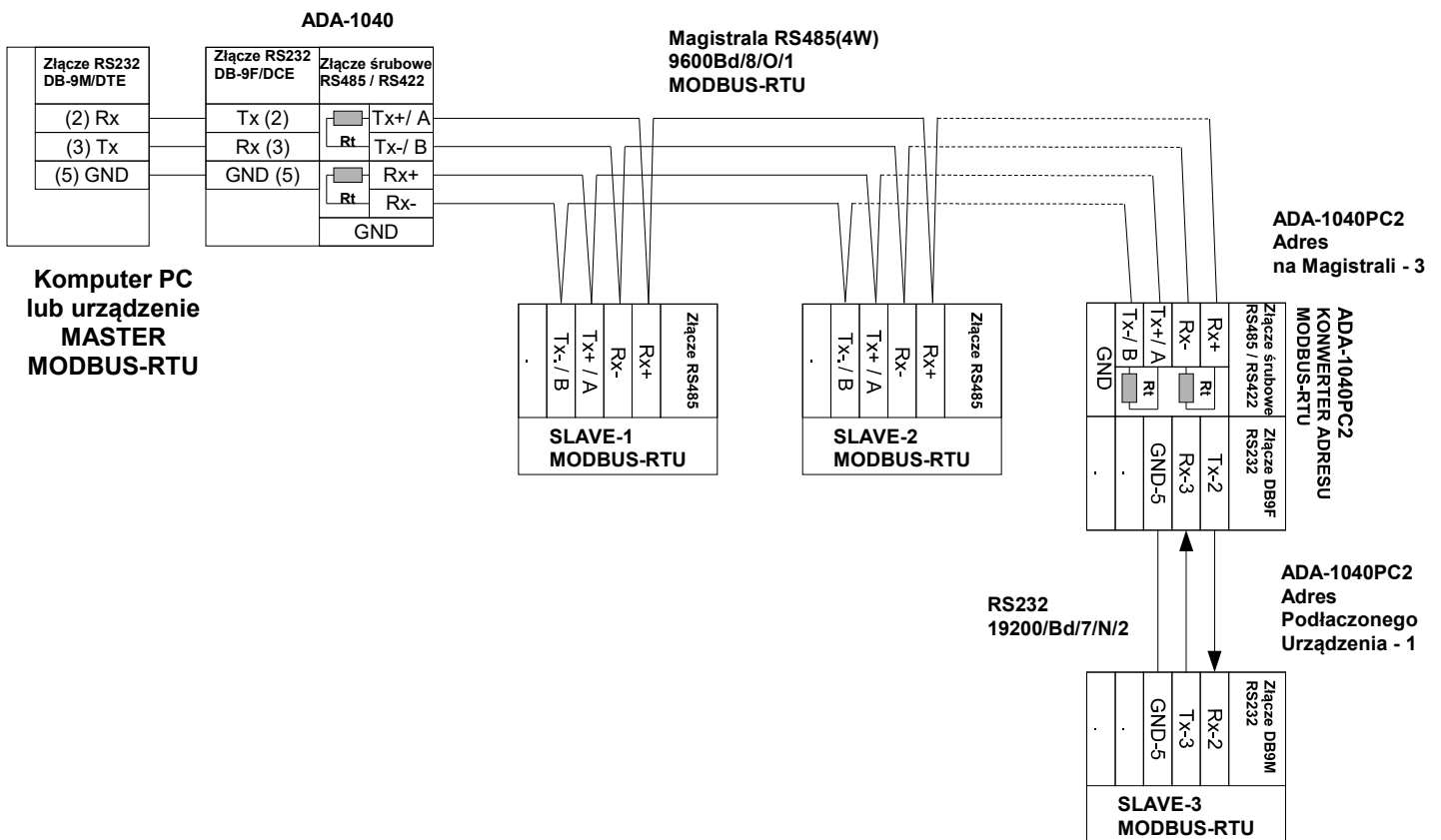
Rys 6. Przykładowe podłączenie ADA-1040PC2 do magistrali RS485(4W) 4-przewodowej oraz separacja galwaniczna urządzeń SLAVE
