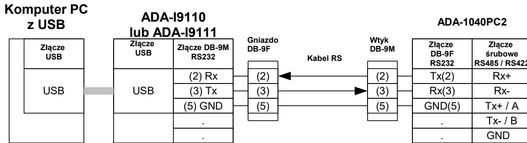
Rys 5. Podłączenie ADA-1040PC2 do komputera PC za pomocą konwertera USB na RS232 ADA-I9110/ADA-I9111
