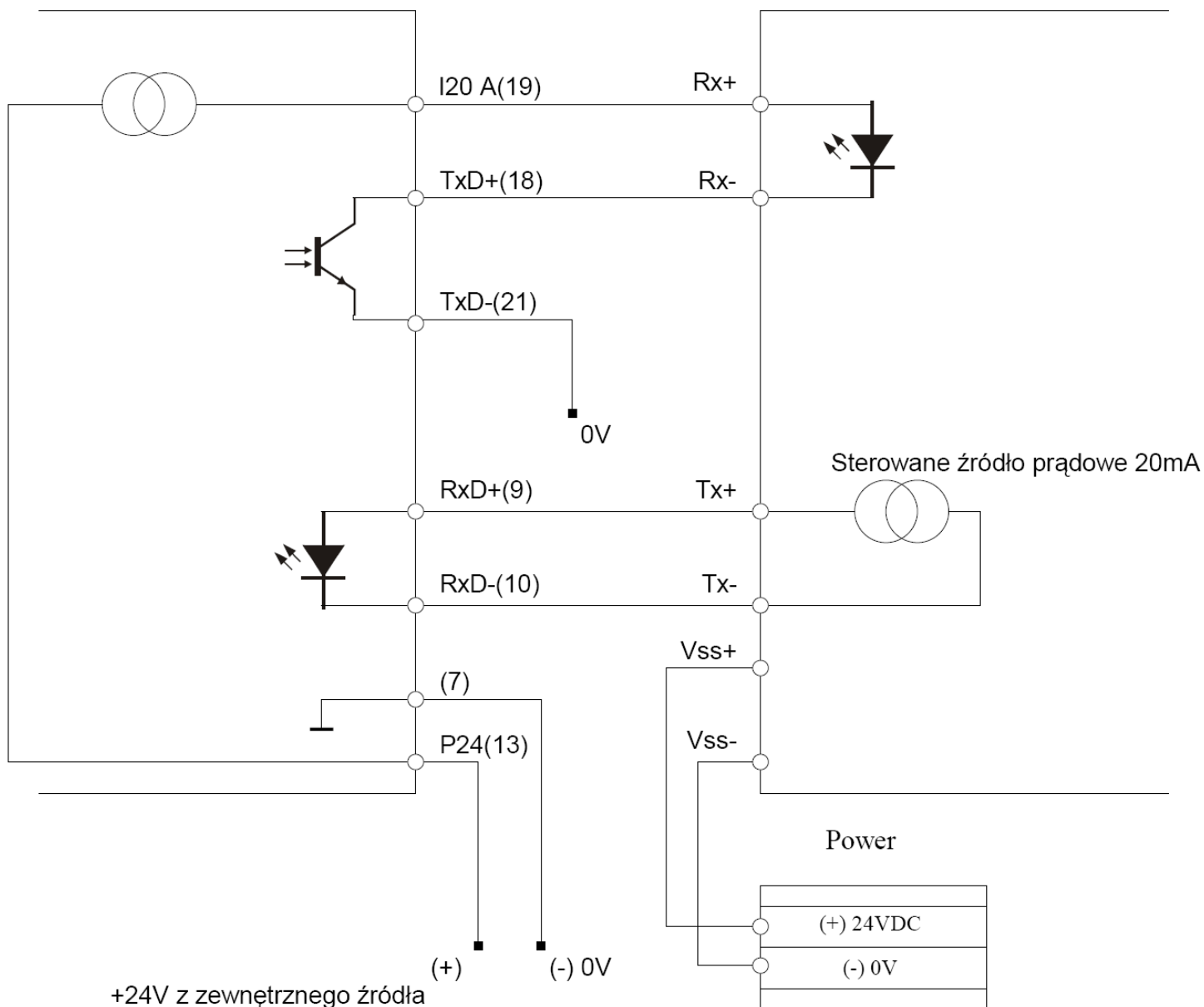
Schemat podłączenia konwertera ADA-1020 do Sterownika SIEMENS S5
