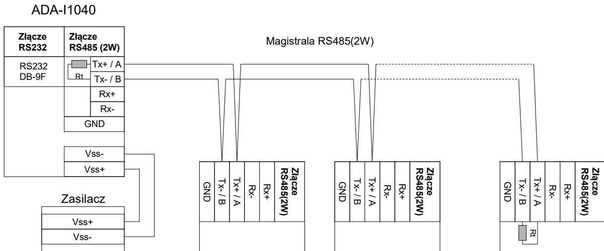
Rys 7. Przykładowe podłączenie urządzeń z interfejsem RS485(2W) do konwertera ADA-I1040
