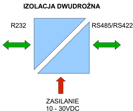
Rys 2. Struktura izolacji w ADA-I1040
