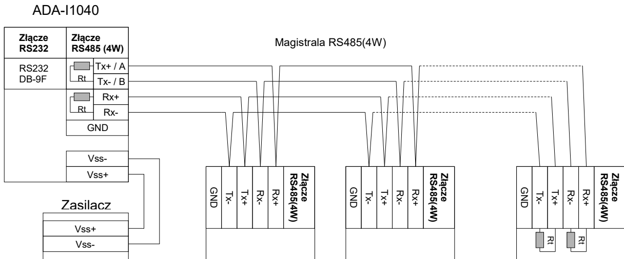
Rys 6. Przykładowe podłączenie urządzeń z interfejsem RS485(4W) do konwertera ADA-I1040
