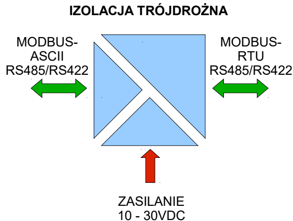
Rys 2. Struktura izolacji
