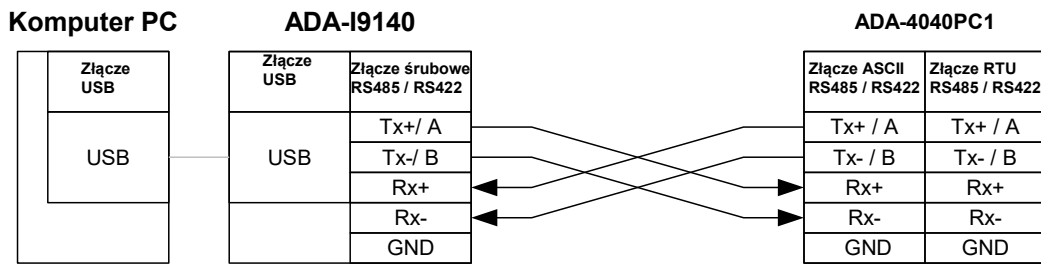
Rys 4. Podłączenie 4-przewodowe ADA-4040PC1 do komputera PC za pomocą konwertera USB na RS485/RS422 ADA-I9140
