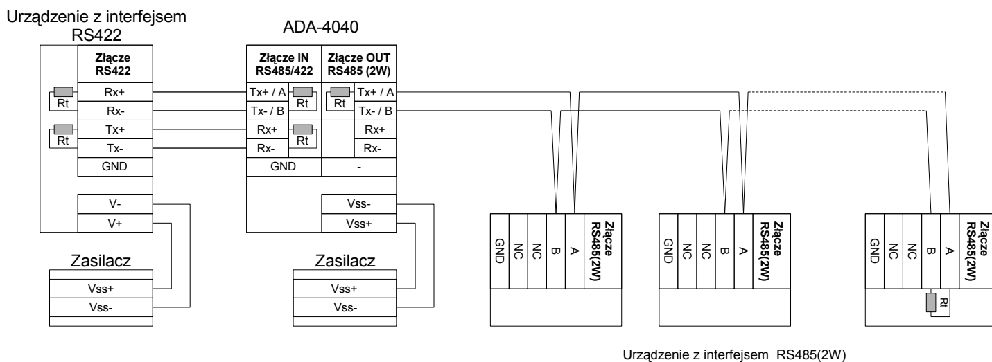
Rys 7. Podłączenie urządzenia z portem RS422 od magistrala RS485(2W) 2-przewodowej
