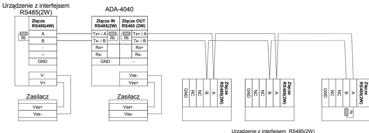
Rys 6. Separacja portu RS485(2W) urządzenia od magistrala RS485(2W) 2-przewodowej
