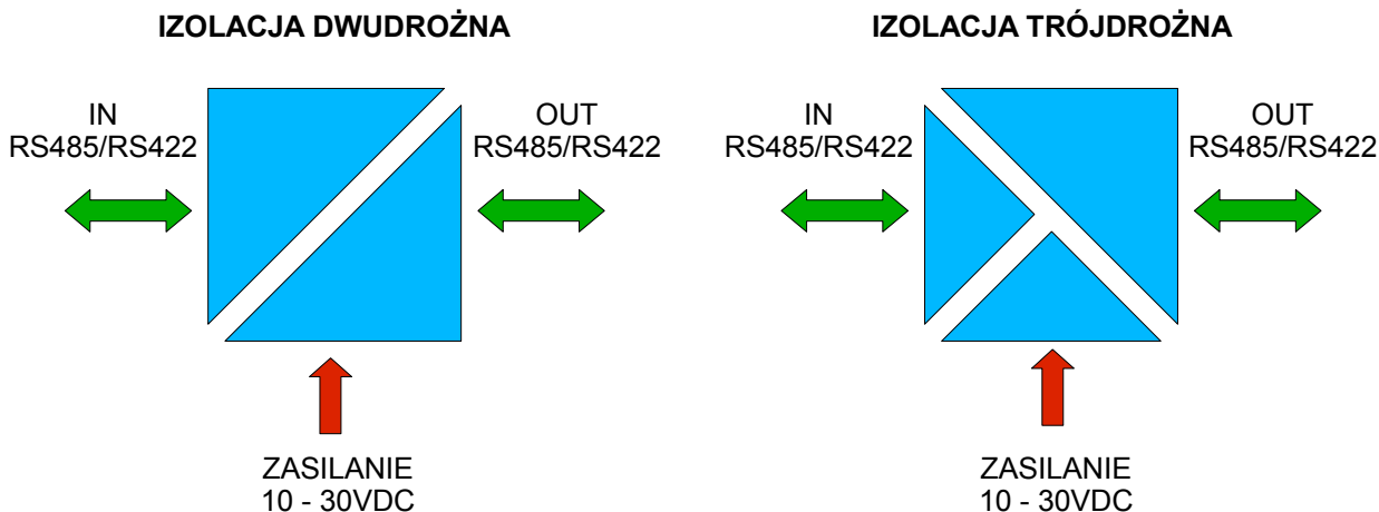
Rys 2. Struktura izolacji
