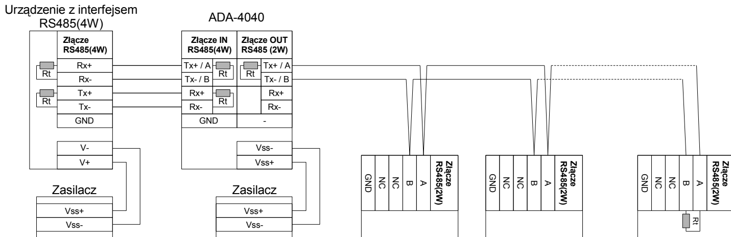
Urządzenie z interfejsem RS485(2W)
