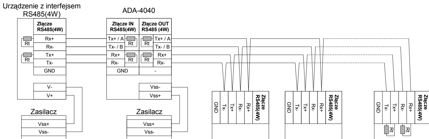
Urządzenia z interfejsem RS485(4W)
