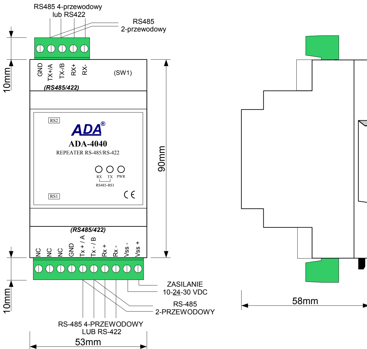
Rys 1. Widok ADA-4040 oraz położenie przełącznika SW1
