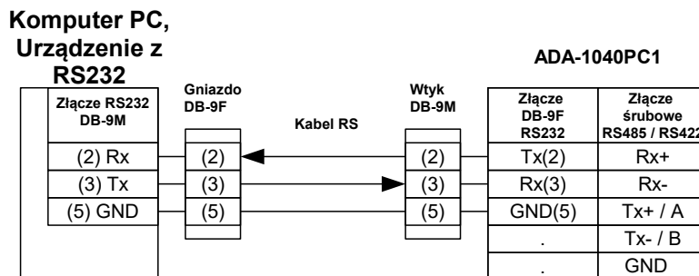
Rys 4. Podłączenie ADA-1040PC1 do komputera PC lub urządzenia z RS232 za pomocą kabla
